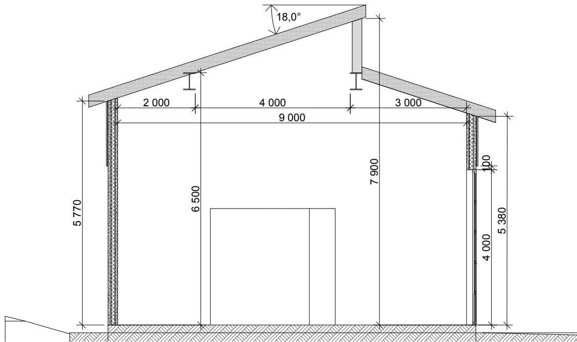
SNITT A-A
