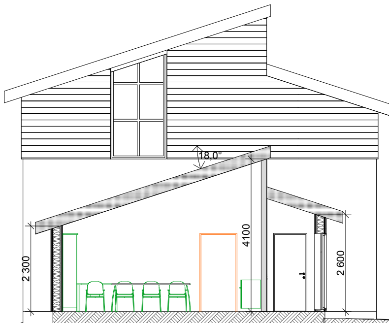
SNITT B-B
